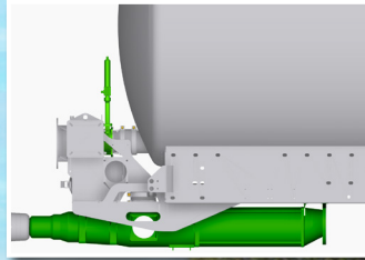
Pompe à colimaçon avec ramasse-pierres et pré-équipement pour Jumbo frontal
