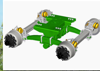
Boggie Roll-Over avec essieu suiveur
