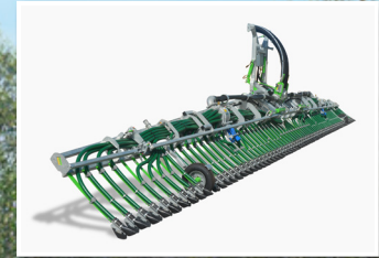
Rampe PENDISLIDE PRO 120/48PS2
